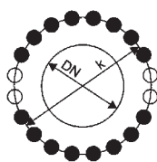
DN 500-600
