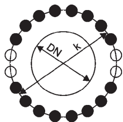
DN 450-600
